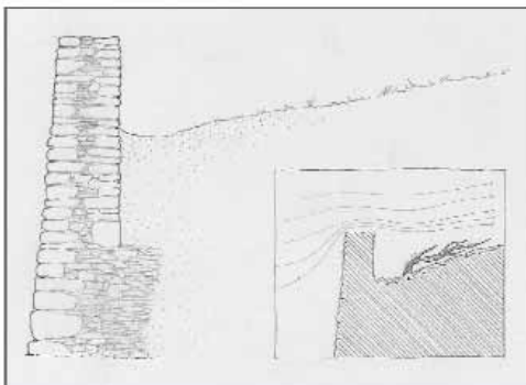
Schema di sezione di un muro a secco con la testa del muro rialzata. La parte di muro rialzata è costituita da un doppio paramento murario. Svolge un ruolo di protezione delle coltivazioni dai venti e di interruzione del flusso delle acque di scorrimento superficiale.
