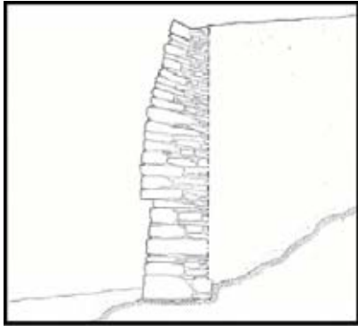
Caso in cui si ha uno scorrimento degli elementi
