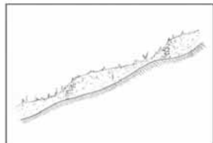
Schema di sezione di un versante sistemato con cigli erbosi.
