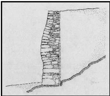
"spanciamento" della parte mediana
