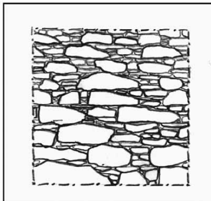
I giunti verticali devono essere sfalsati nei diversi strati di pietre.
