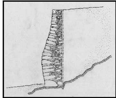
"spanciamento" della parte inferiore
