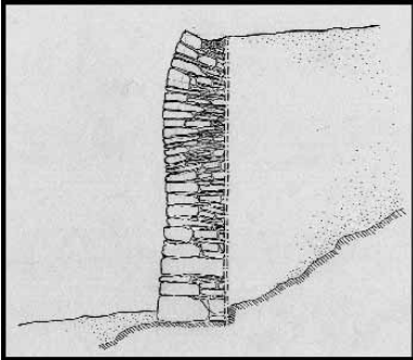
"spanciamento" della parte superiore
